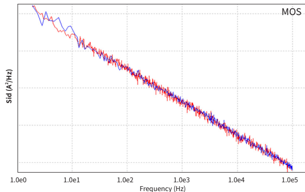
1/f 噪声，Drain 端电流功率谱
