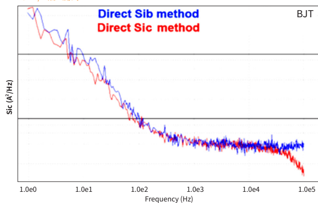
BJT 1/f 噪声测试
