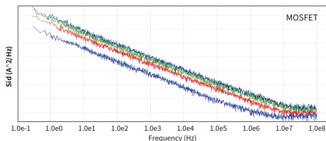
1/f 噪声测试, 100MHz 带宽
