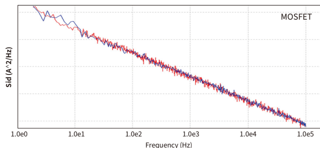
1/f 噪声测试, 电流功率谱
