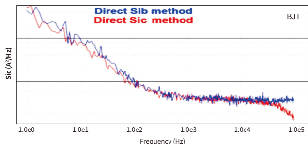
1/f 噪声测试
