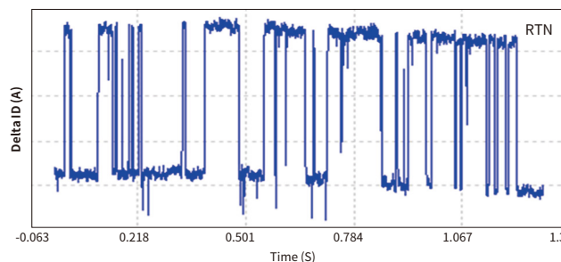
RTN 噪声测试
