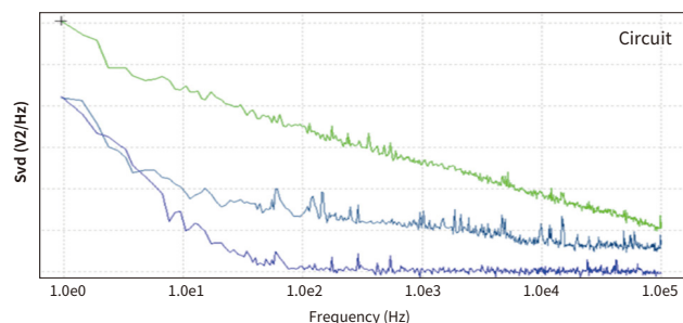
1/f 噪声测试, 电压功率谱
