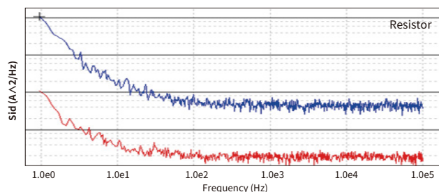
热噪声测试
